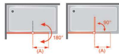
Dibujo técnico VI425
