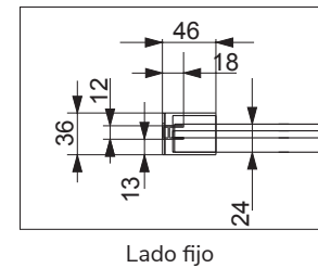
Dibujo técnico GS607 + GS607 Angular de Ducha
