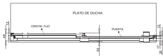
Dibujo técnico VO102 Frente de Ducha con perfil de cierre
