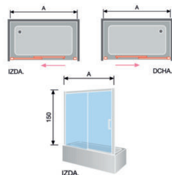
Dibujo técnico SU152 Frente de ducha
