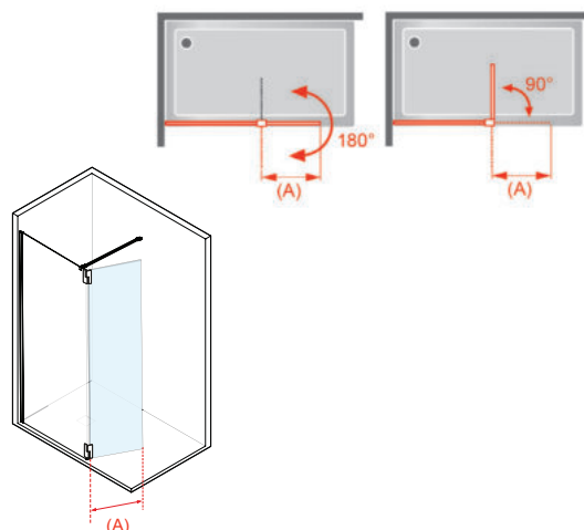
Dibujo técnico VI425
