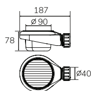
Válvula Viega (opcional) 22HCRAHVAS002001
