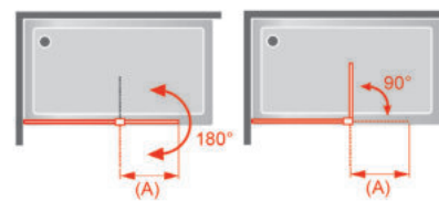
Dibujo técnico VI525
