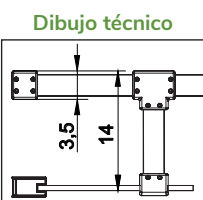
Detalle fijación barra a pared
