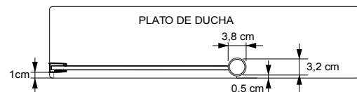
Dibujos técnicos FL633 Panel Fijo de Ducha a Techo
