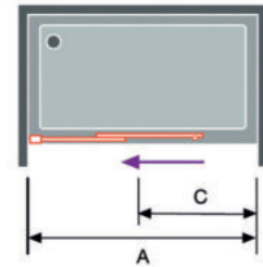
Dibujo técnico GS102 Fronte de Ducha
