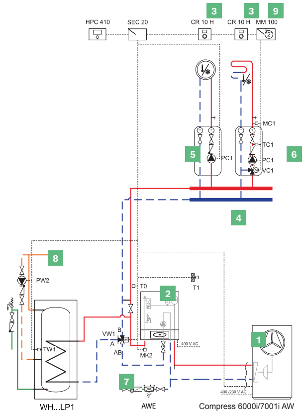
Esquema de instalación AWE (resistencia)
