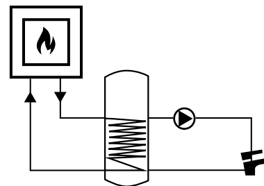
Acumulador
